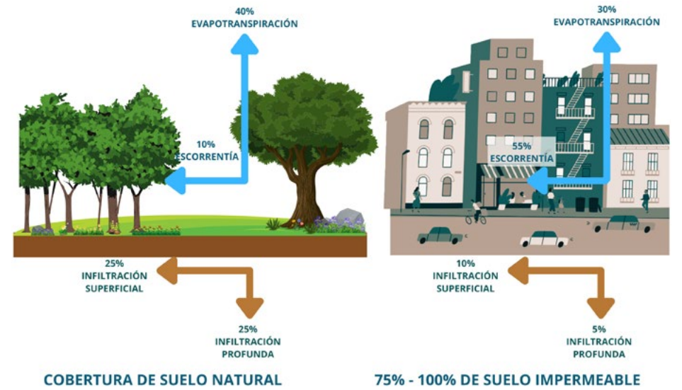
Figura 8. Capacidad de infiltración en ciudades.
